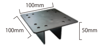
ダウン島設置用パーツ(2Way土台用)
